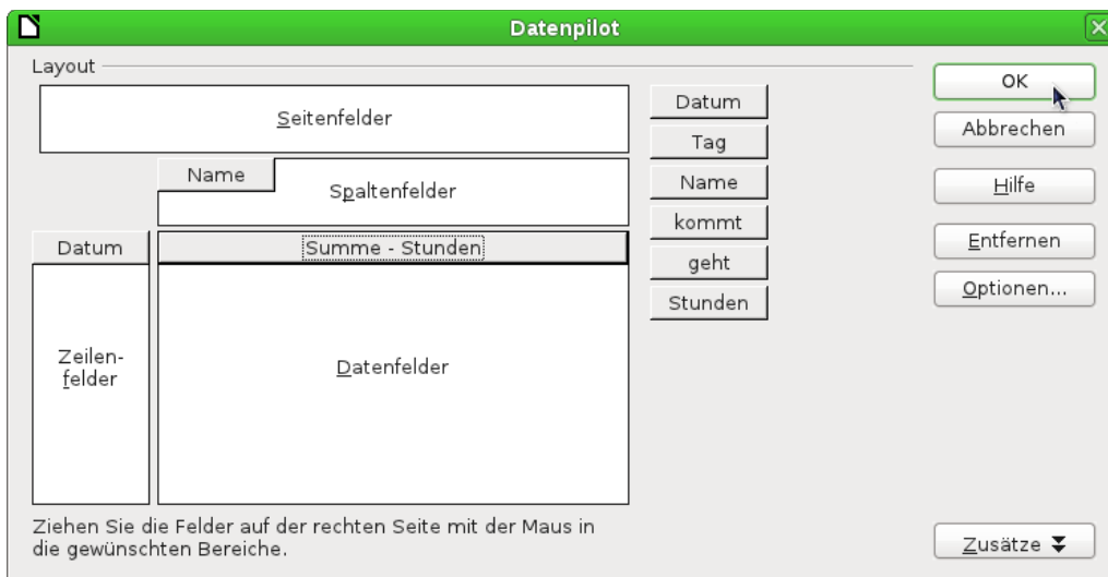
Abbildung 2: Dialog Datenpilot
