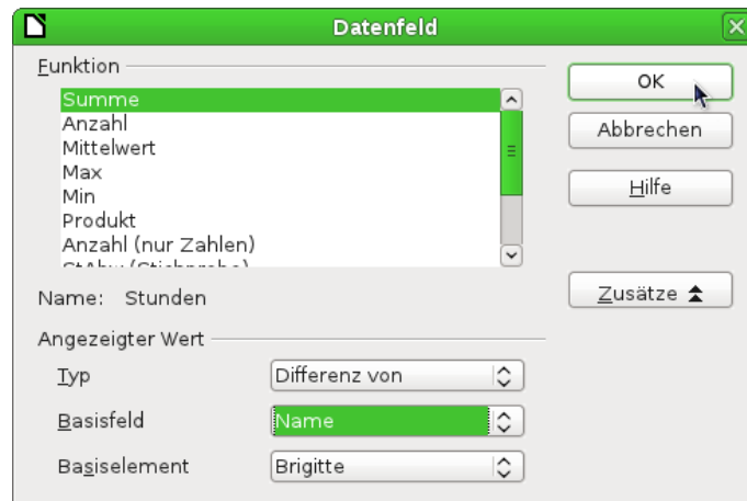
Abbildung 4: Datenfeld
